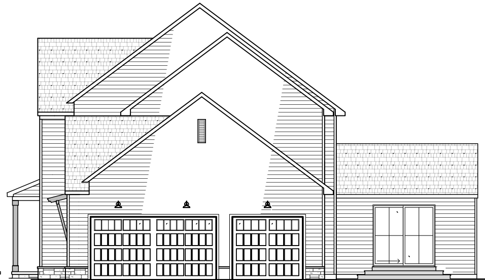
RIGHT ELEVATION
